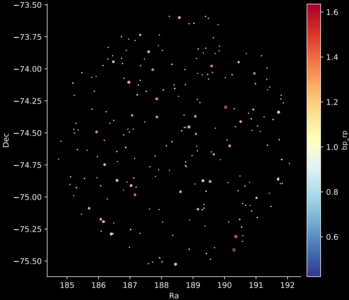
GALAH DR4 Field: [7173] Stars: 220
