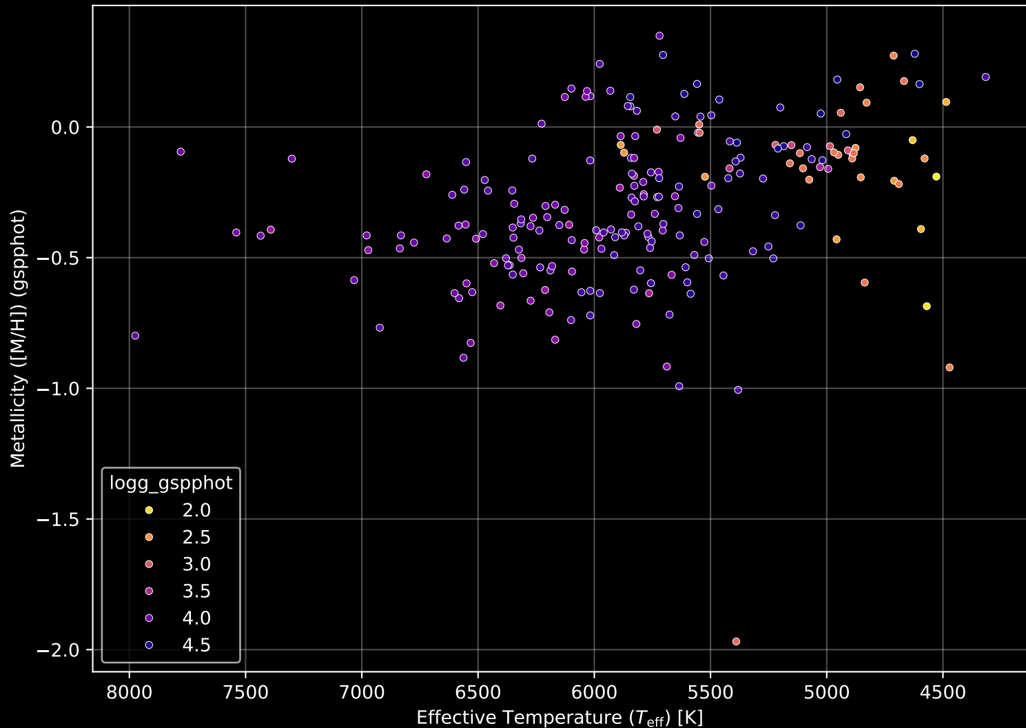
GALAH DR4 Field: [7173] Stellar Population Parameters (n= 220)
